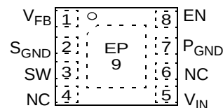
MCP1662 2x3 TDFN*
